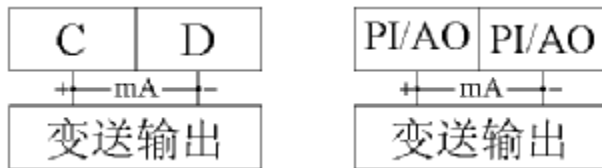
图 7 模拟量输出信号接线图
