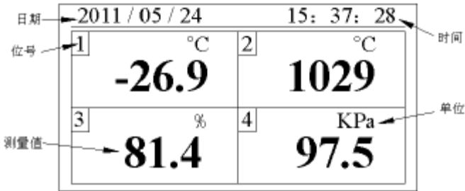
图10 总貌画面
