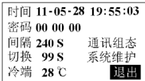
图 21 系统组态画面
