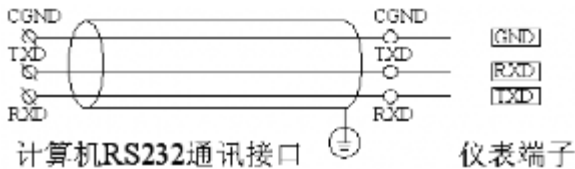
图 27 RS-232 通讯接线方法
