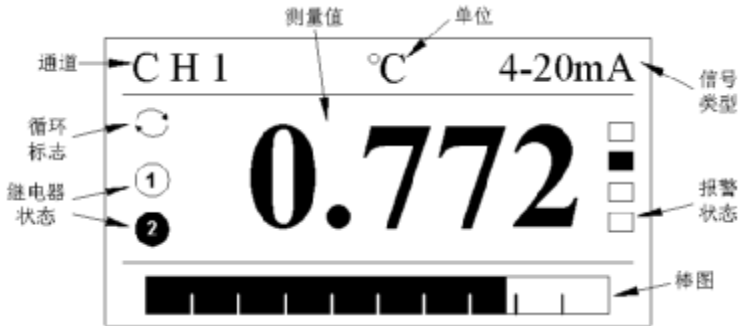
图11 数显画面
