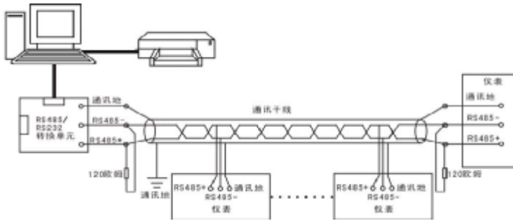
图 28 RS-485 通讯接线方法
