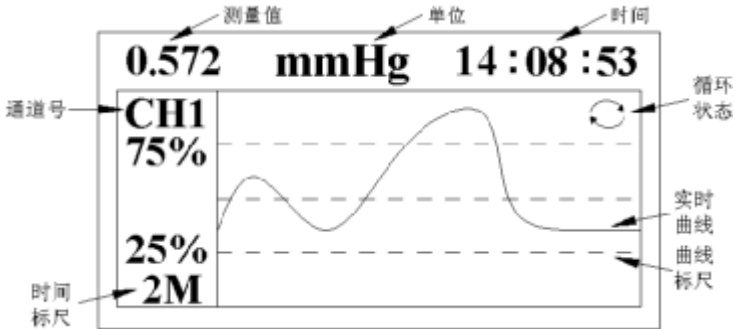
图12 实时趋势画面
