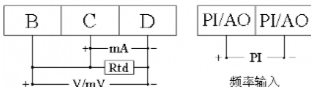
图4 模拟量、频率输入信号接线图
