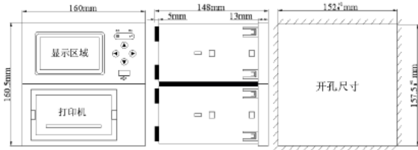
图1 仪表尺寸
