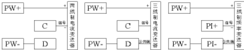
图 6 变送器电源输出接线图
